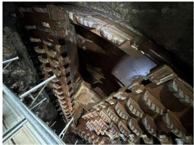
羊蹄トンネル(比羅夫)(ニセコ町・倶知安町) 中間立杭マシン面板
